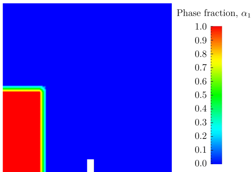
図 2.21 相比率 alpha1 の初期条件
