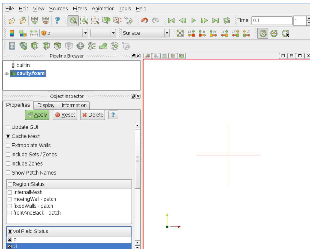
図 6.1 paraFoam の画面
