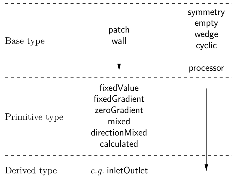
図 5.2 境界タイプの階層
