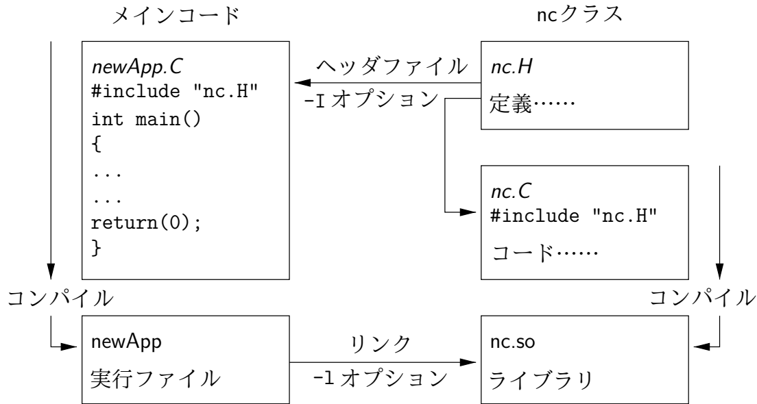
図 3.1 ヘッダファイル，ソースファイル，コンパイル，リンク
